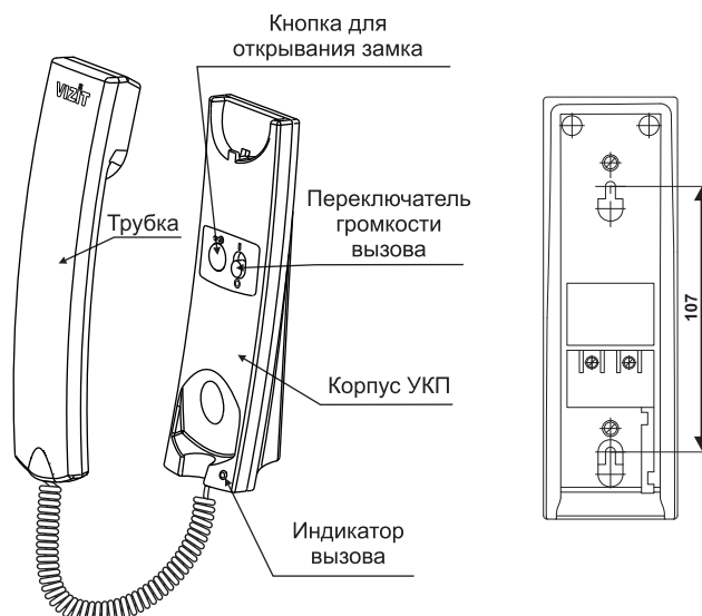
Рисунок 1 - Расположение органов управления и установочный размер
